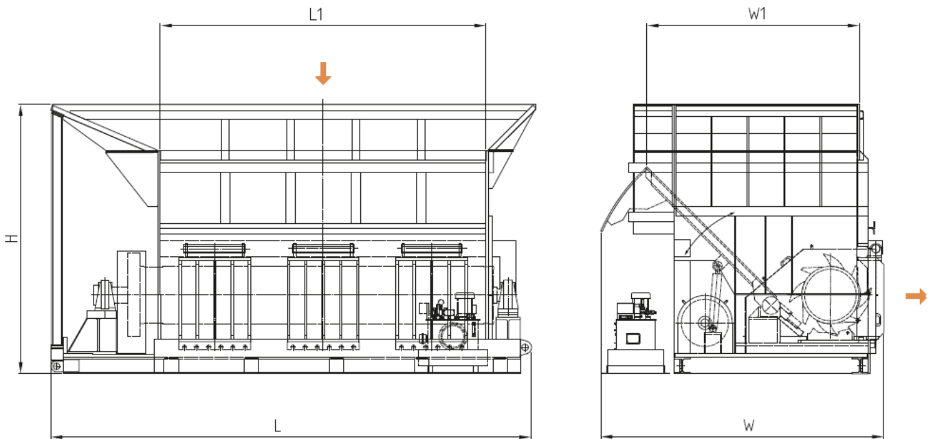
Technische Zeichnung Großbrecher
